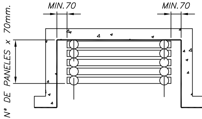
DIMENSIONES DE UN PANEL SIMPLE
