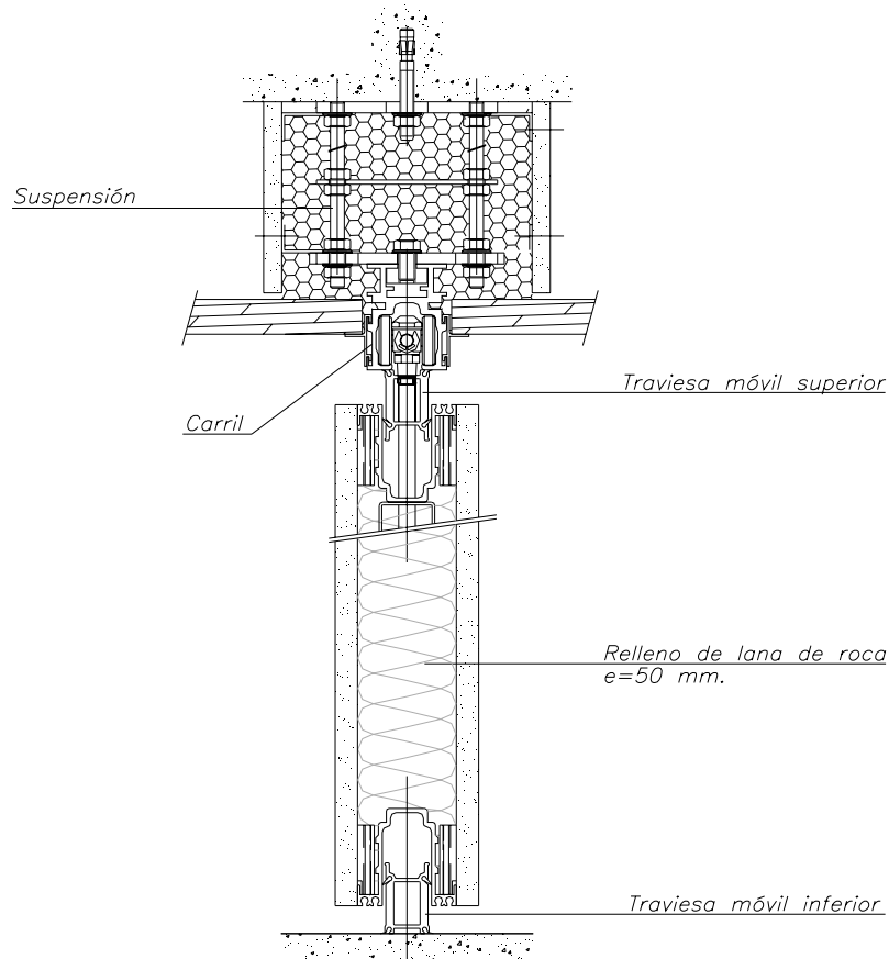
Sección Vertical REITER 1900
