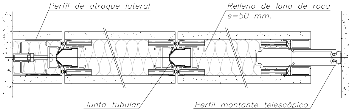
Sección Horizontal REITER 1900
