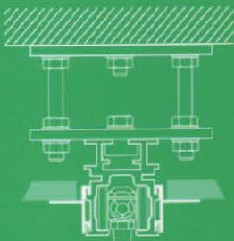
Carril Monodireccional Montaje: Falso techo
