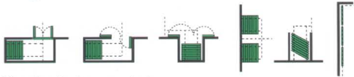
Ejemplos de almacenamiento de los Tabiques Móviles Multidireccionales
