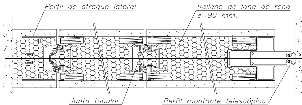
Sección Horizontal HUF COR 8701
