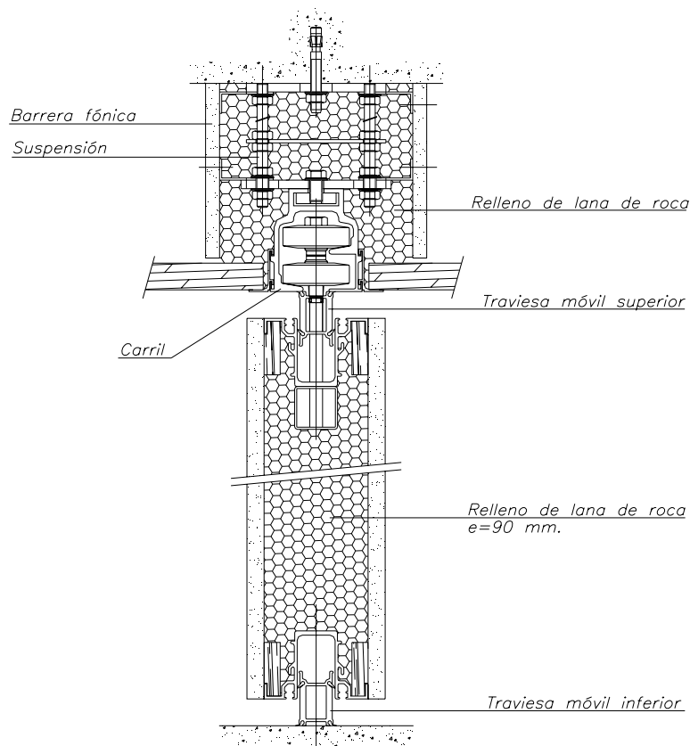
Sección Vertical HUF COR 8701
