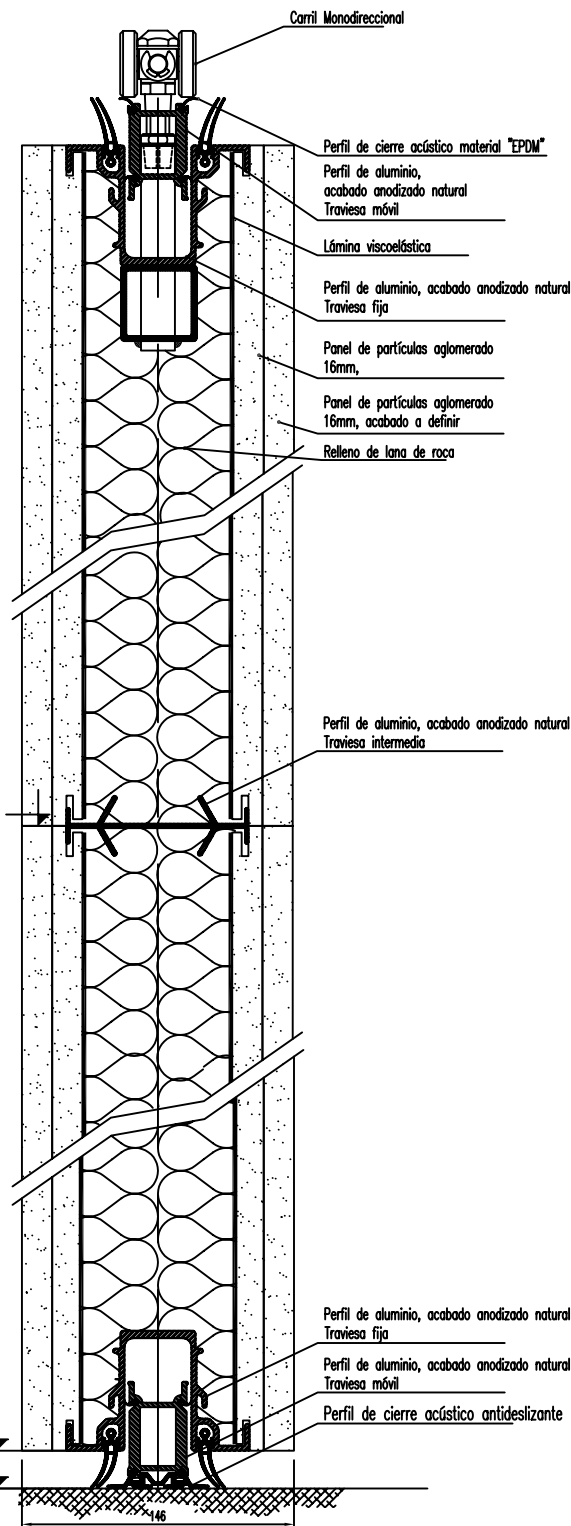
SECCION VERTICAL
