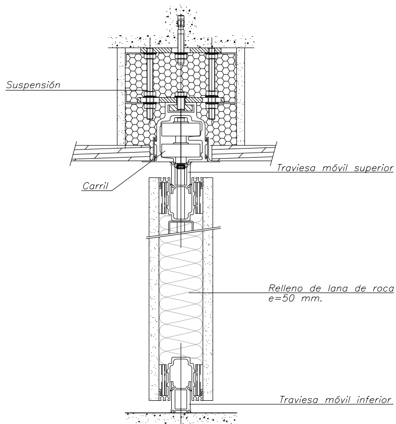
Sección Vertical HUF COR 8601
