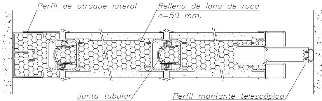
Sección Horizontal HUF COR 8601
